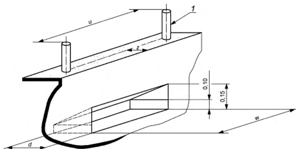
1 — поручень, d — расстояние между центральной линией ступени и вертикальной поверхностью; w — ширина ступени; u — расстояние между параллельными поручнями, между которыми должен быть обеспечен проход; z — расстояние между ступенью и поручнем/перилами
