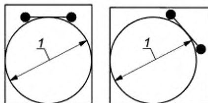
1 — внутренний диаметр ограждения
